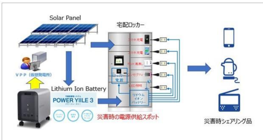
「シェアリング防災宅配ロッカー」概要図
